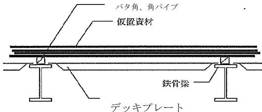
図-1 資材仮置き方法(S造の場合)
