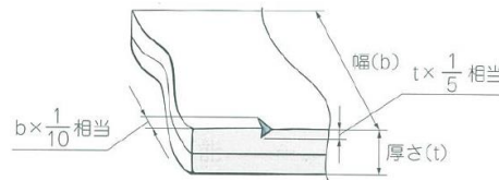
(b) 幅方向、厚さ方向の傷の判定基準
