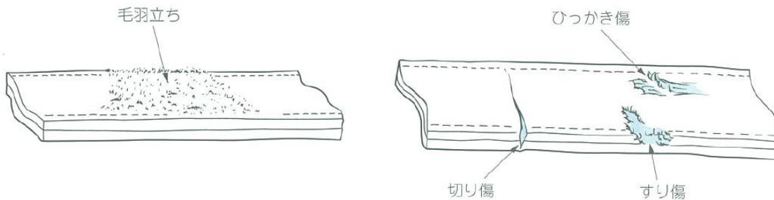
(a) ベルトスリングの損傷例
