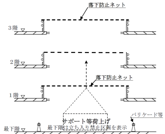
断面
