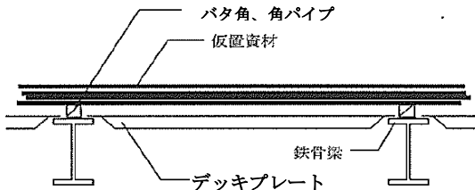
図-1 資材仮置き方法(S造の場合)
